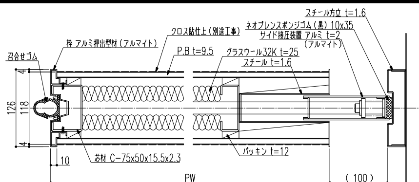
ASD-S120B 横断面図 ; サイド装置付パネル (SP)
