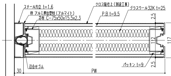
ASD-S100A 横断面図 ; 一般パネル(NP)
