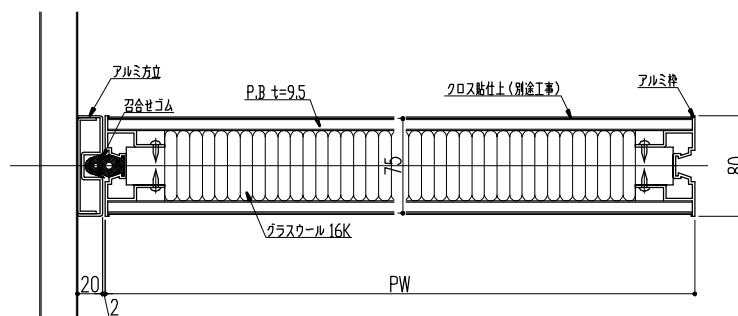
ASD-S80A 横断面図 ; 一般パネル (NP)
