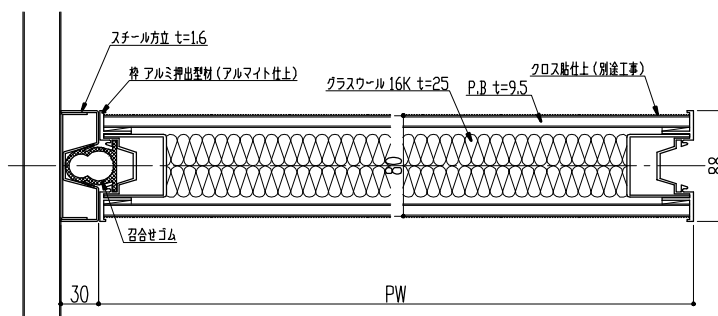
ASD-S90A 横断面図 ; 一般パネル (NP)
