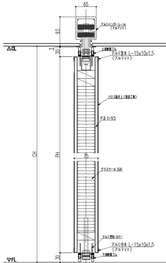
ASD-S80A 立断面図 ; 一般パネル (NP)
