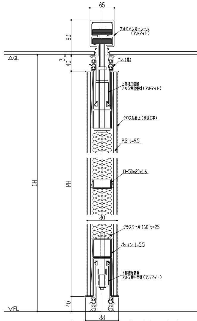
ASD-S90A 立断面図 ; 一般パネル (NP)
