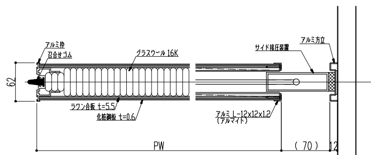
ASD-S60B 横断面図 ; サイド装置付パネル (SP)
