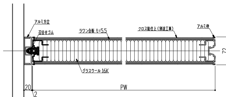
ASD-S70A 横断面図 ; 一般パネル (NP)
