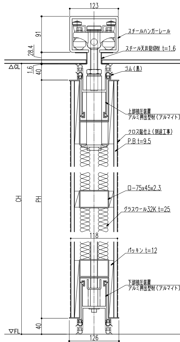
ASD-S120B 立断面図 ; 一般パネル (NP)
