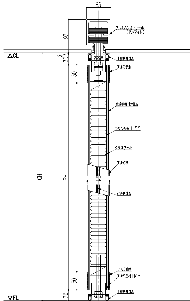
ASD-S60B 立断面図 ; 一般パネル (NP)
