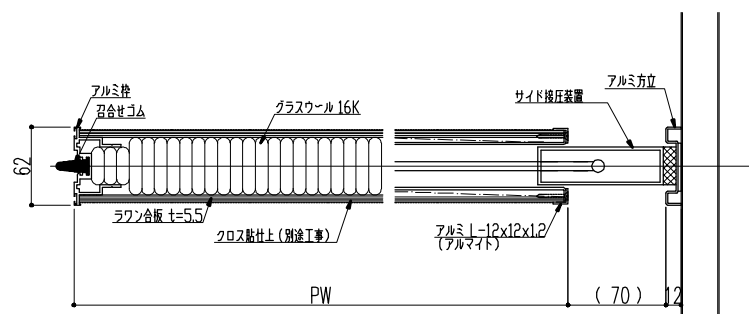
ASD-S60A 横断面図 ; サイド装置付パネル (SP)
