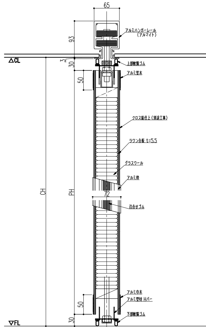
ASD-S70A 立断面図 ; 一般パネル (NP)
