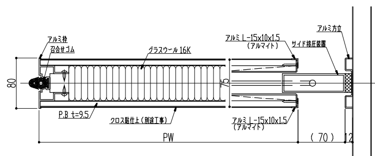
ASD-S80A 横断面図 ; サイド装置付パネル (SP)
