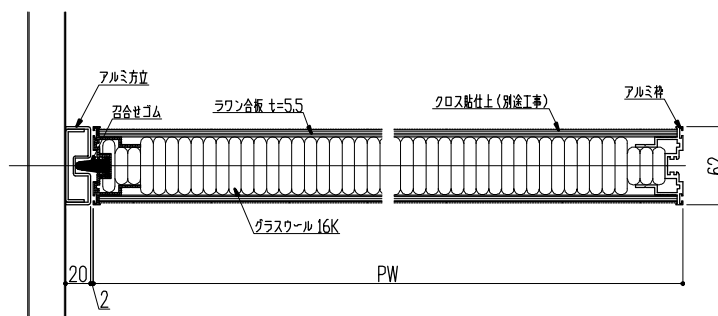
ASD-S60A 横断面図 ; 一般パネル (NP)
