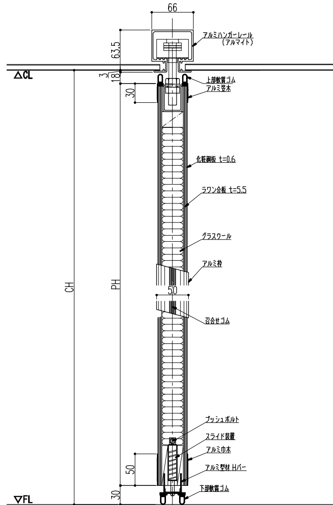
ASD-S50B 立断面図 ; 一般パネル (NP)
