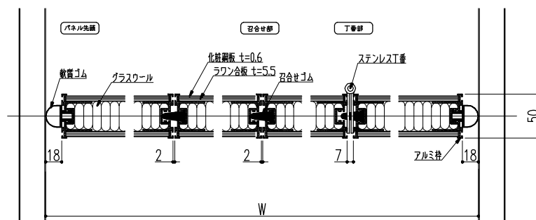
ASD-S50B 横断面図 ; 小扉タイプ
