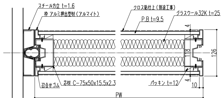
ASD-S120B 横断面図 ; 一般パネル (NP)
