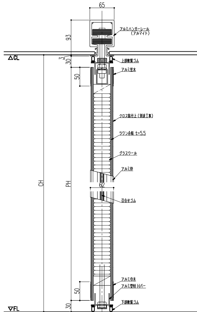
ASD-S60A 立断面図 ; 一般パネル (NP)
