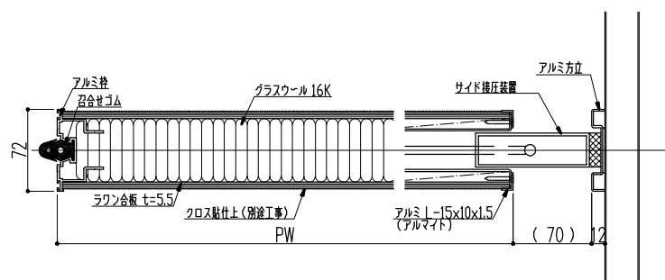
ASD-S70A 横断面図 ; サイド装置付パネル (SP)
