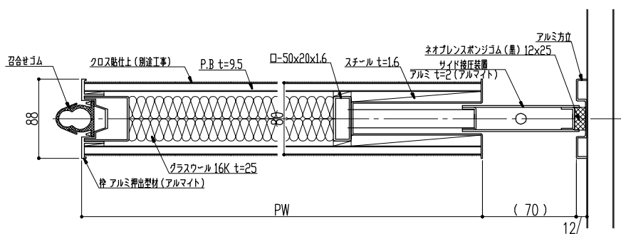
ASD-S90A 横断面図 ; サイド装置付パネル (SP)
