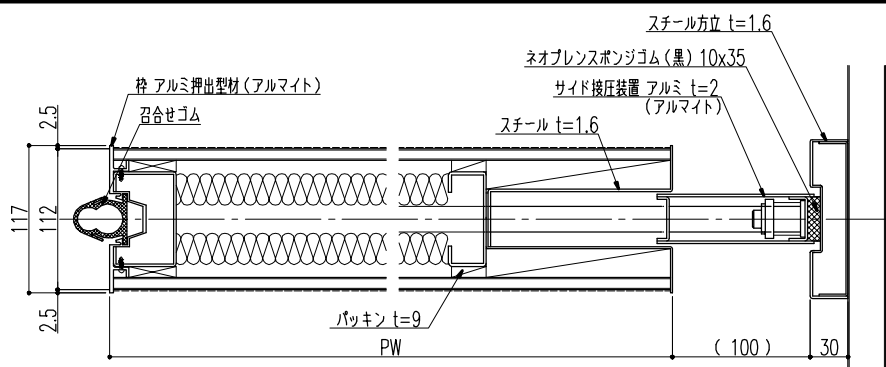
ASD-S100A 横断面図 ; サイド装置付パネル(SP)
