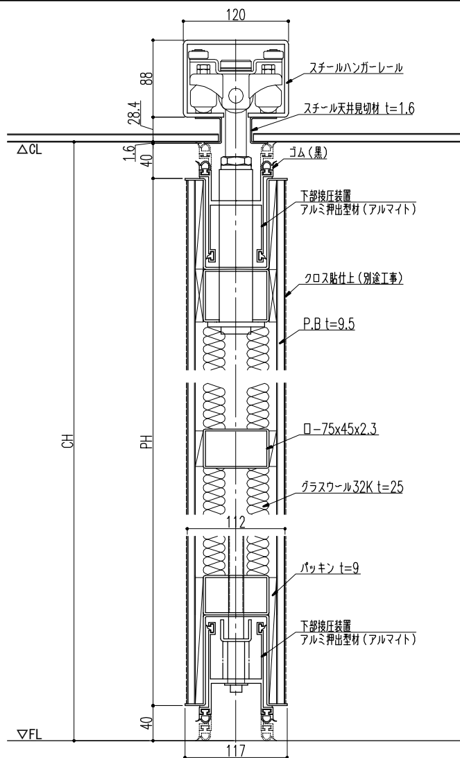
ASD-S100A 立断面図 ; 一般パネル(NP)
