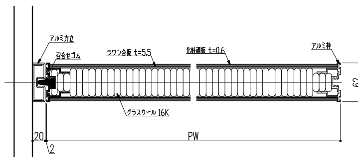
ASD-S60B 横断面図 ; 一般パネル (NP)
