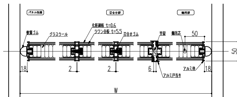
ASD-S50B 横断面図 ; 軸吊タイプ
